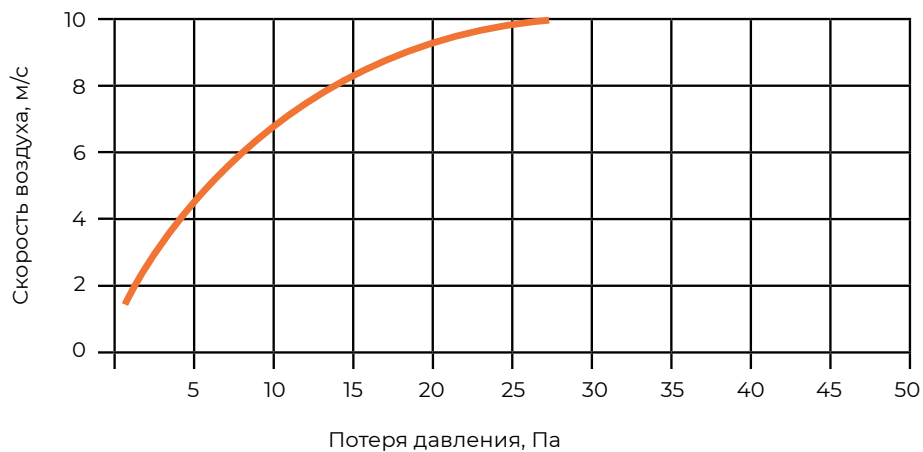
Диаграмма падения давления в жалюзи HP100
