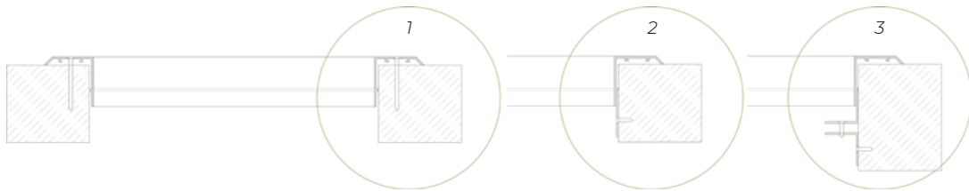
Габаритно-посадочные размеры фасадной решетки HP100 AxB – размеры строительного проема
